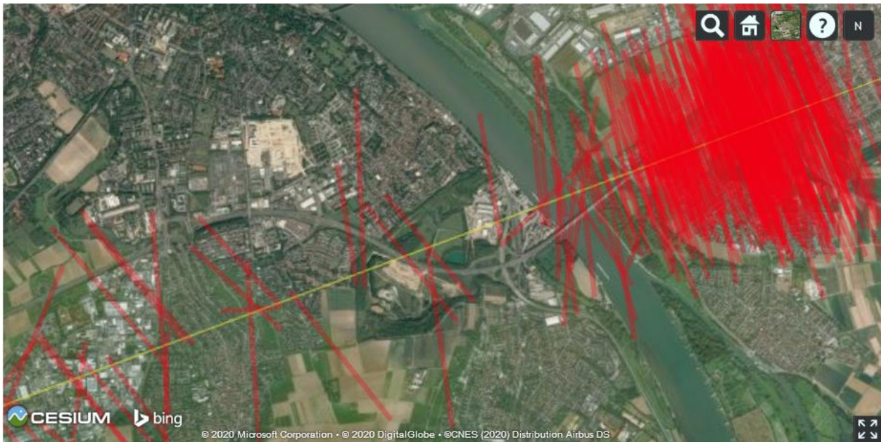
Abb. 5: BR18 & BR25 - Identifizierte Abflüge im September 2019, Draufsicht (Quelle: Bing Maps)
