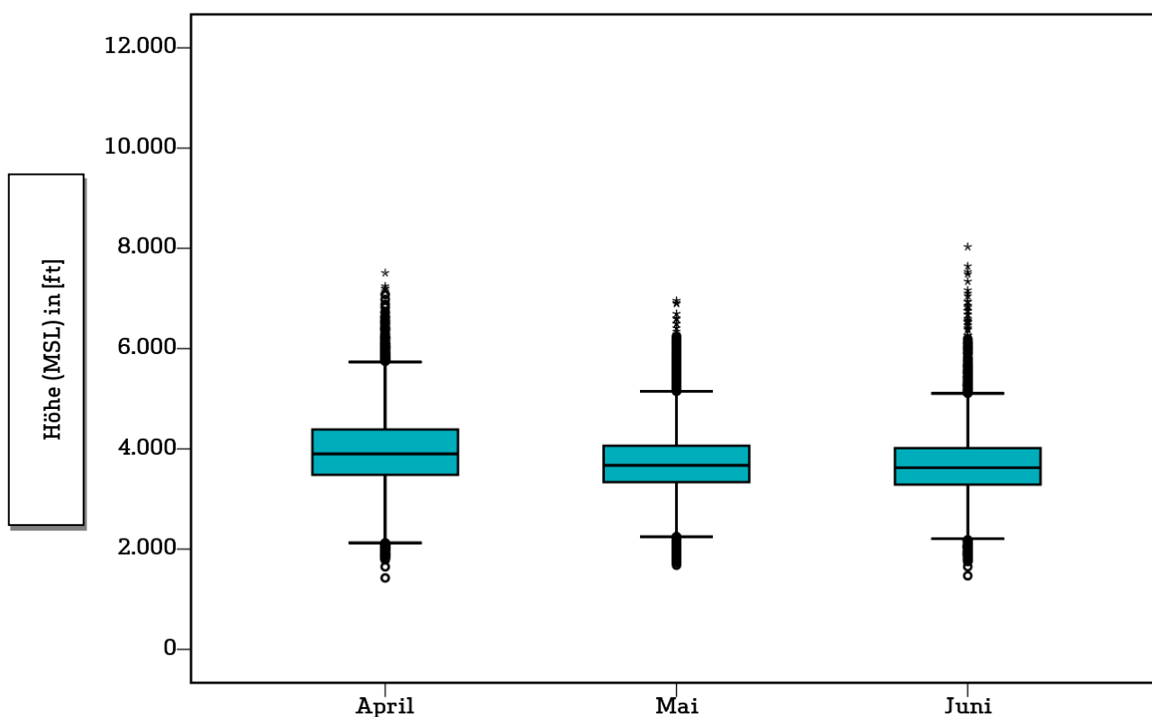
Abb. 4: Boxplots - Abflughöhen bei Betriebsrichtung 18 und 25
