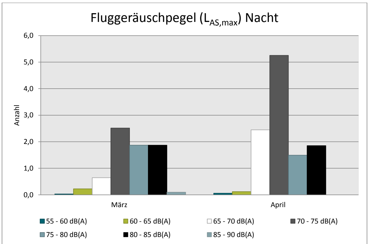
Abb. 9: Tages durchschnitt - Maximalpegelverteilung in der Nacht (Fluggeräusch)
