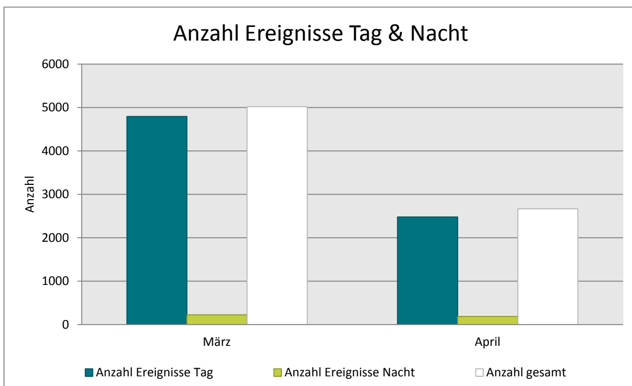
Abb. 7: Anzahl Fluggeräuschereignisse (Tag und Nacht)
