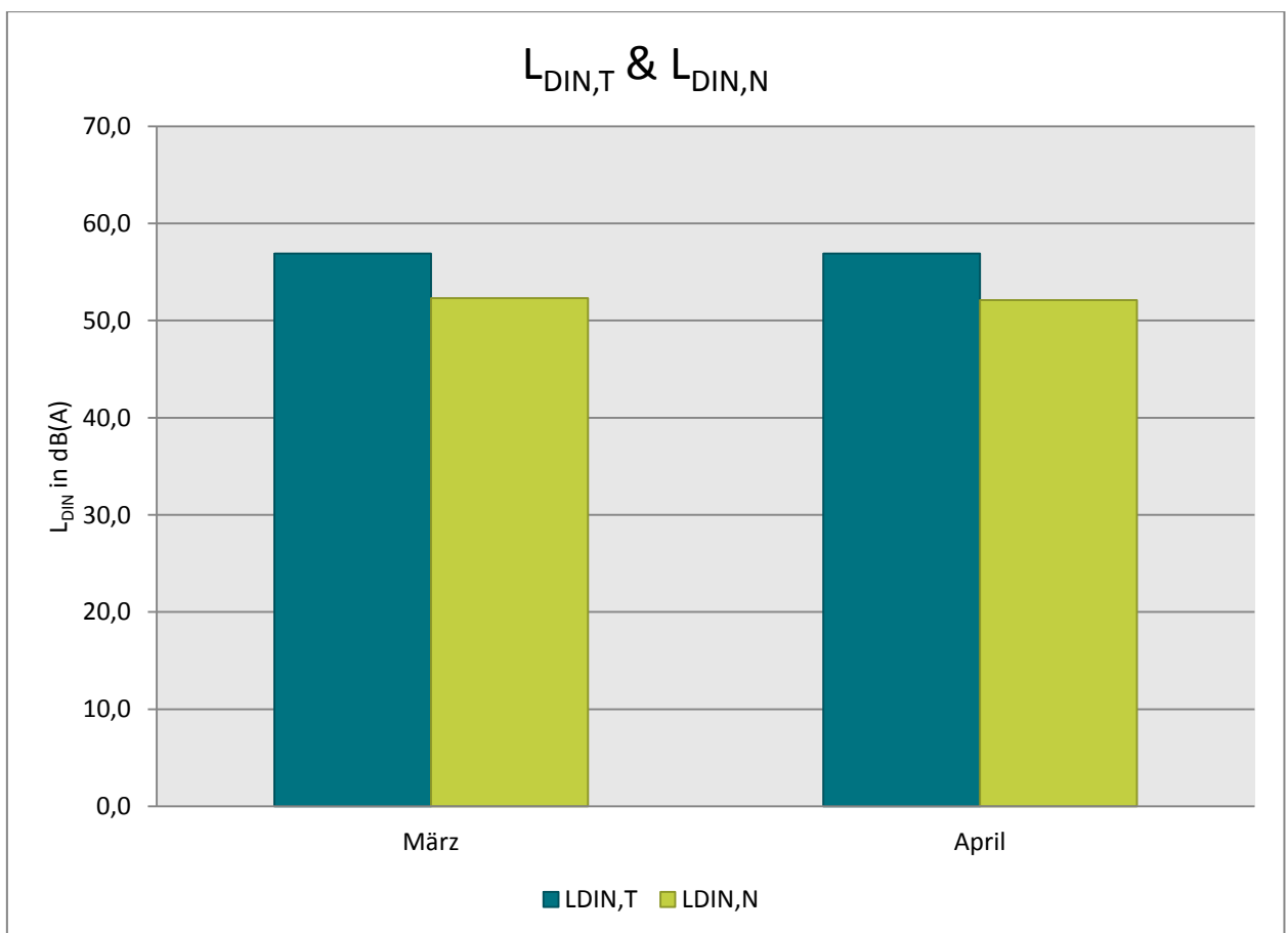
Abb. 10: L_{DIN} Tag und Nacht
