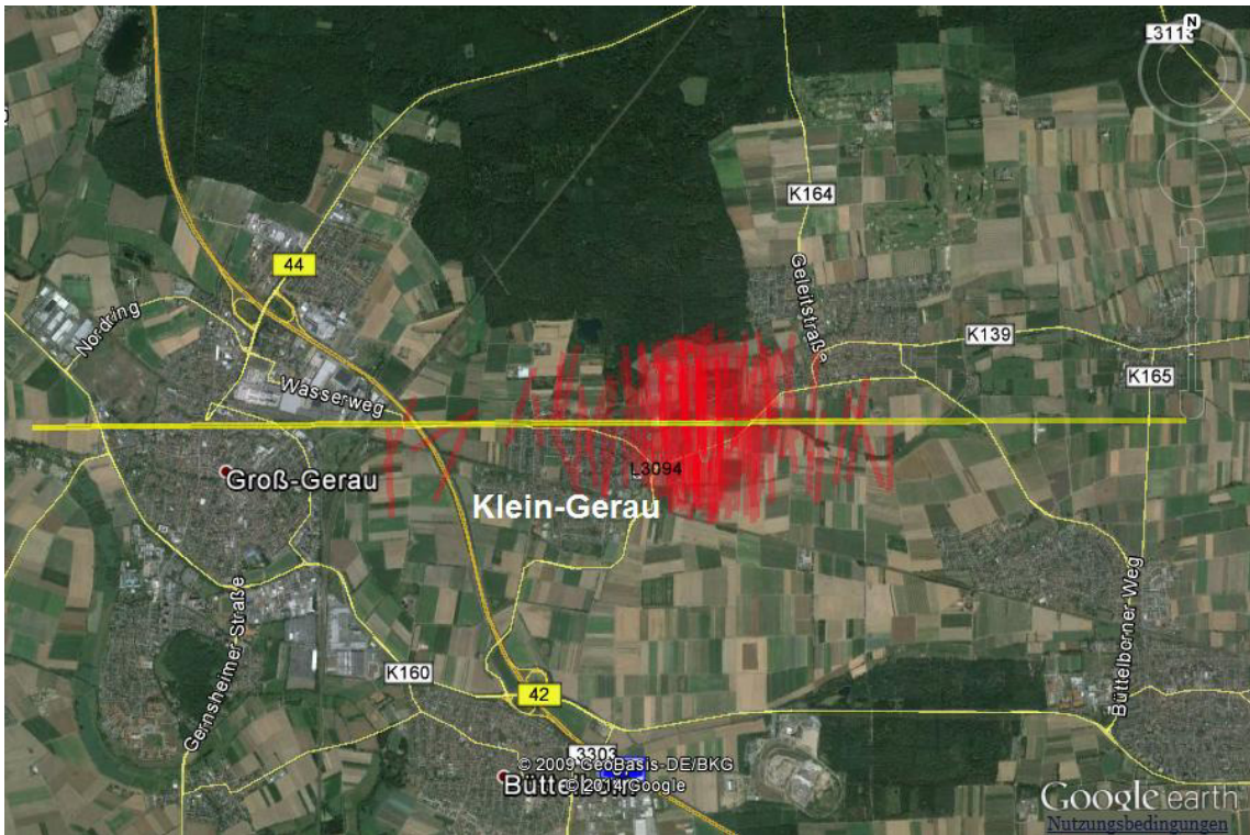
Abb. 3: BR25 & BR18 - Identifizierte Abflüge im April 2013, Draufsicht (Quelle: Google Earth)
