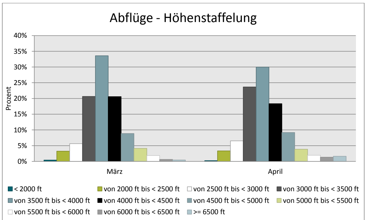
Abb. 6: Prozentualer Anteil der Abflughöhenstaffelung bei Betriebsrichtung 25 & 18
