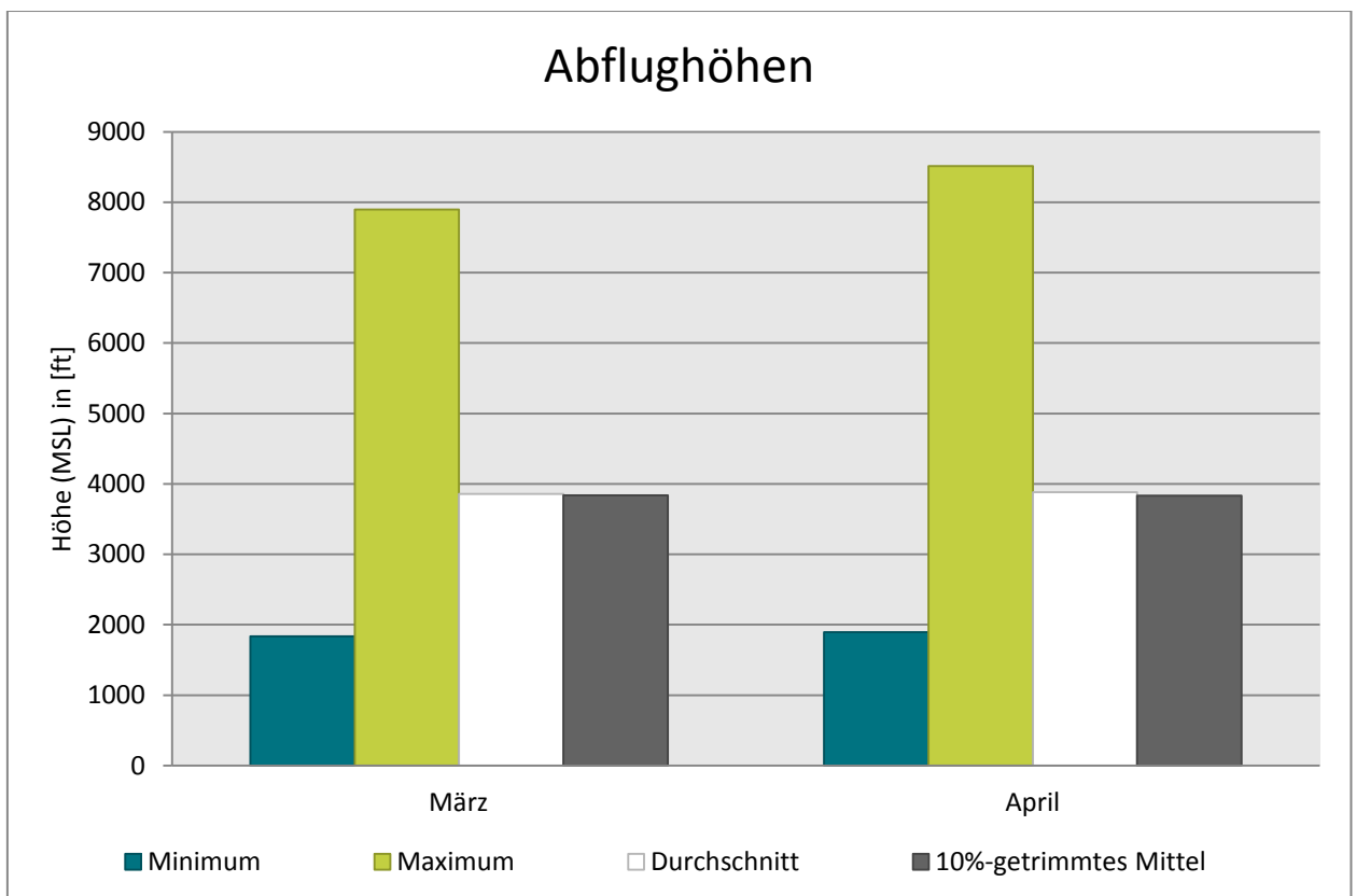
Abb. 4: Abflughöhen bei Betriebsrichtung 25 & 18
