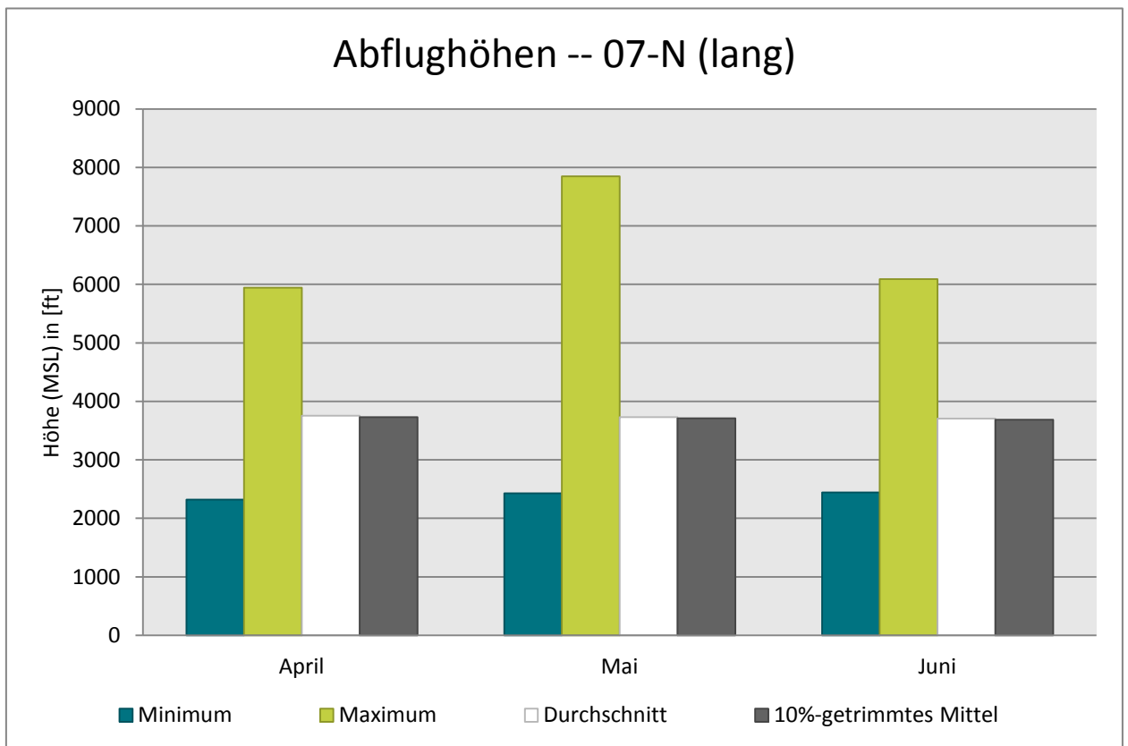
Abb. 10: Abflughöhen bei Betriebsrichtung 07 -- Abflugroute 07-N (lang)
