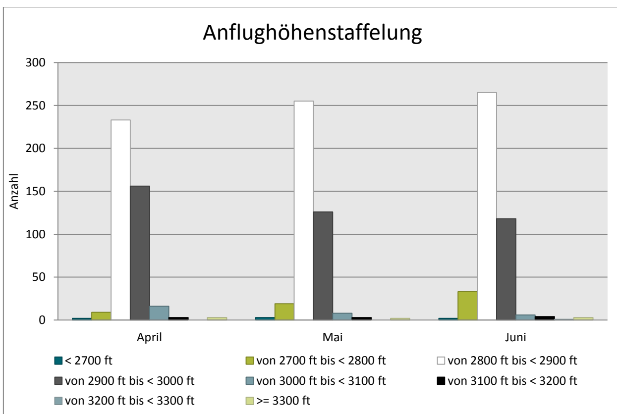
Abb. 9: Anflughöhenstaffelung bei Betriebsrichtung 25
