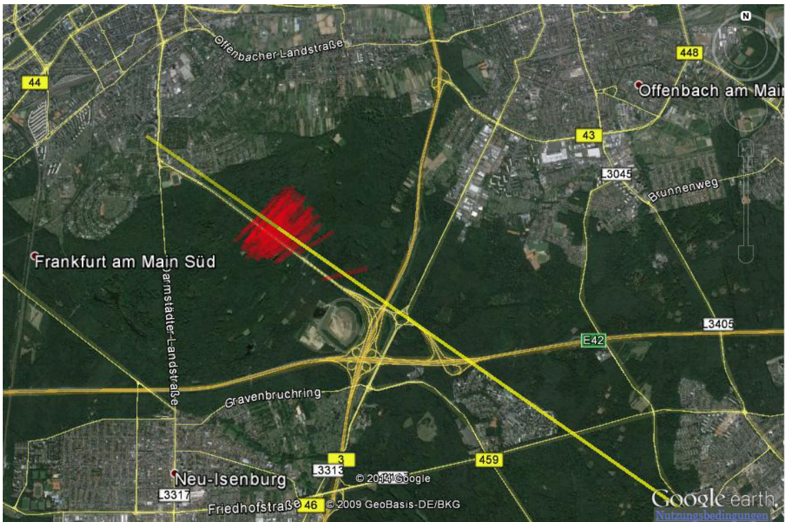
Abb. 5: BR07 (07-N lang) - Identifizierte Abflüge im Juni 2014, Draufsicht (Quelle: Google Earth)
