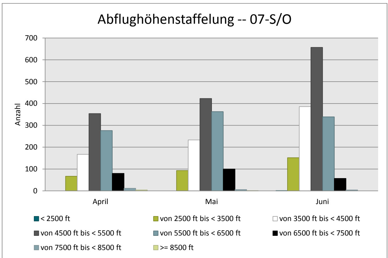
Abb. 13: Abflughöhenstaffelung bei Betriebsrichtung 07 -- Abflugroute 07-S/O
