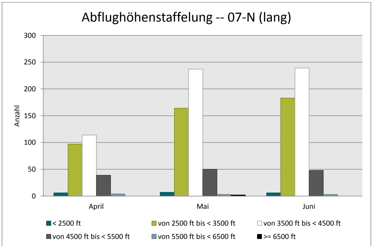
Abb. 11: Abflughöhenstaffelung bei Betriebsrichtung 07 -- Abflugroute 07-N (lang)
