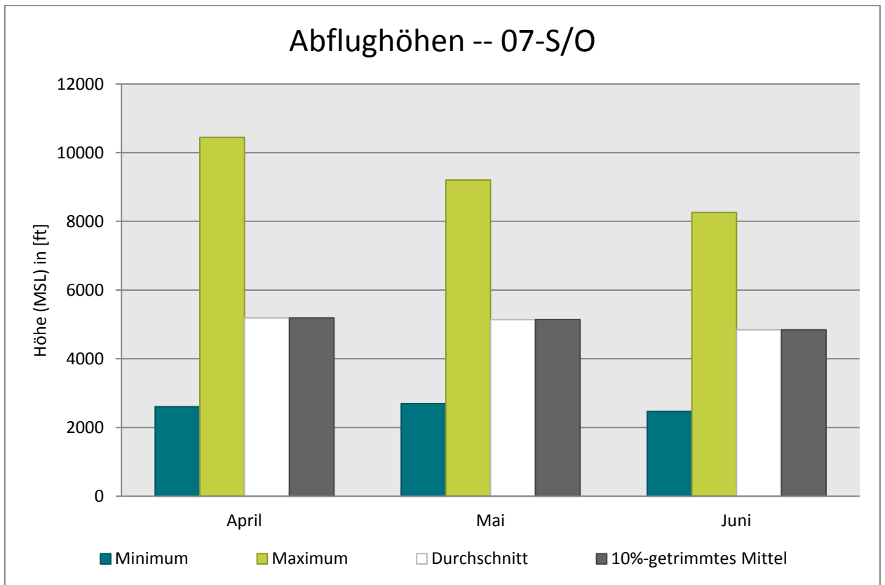
Abb. 12: Abflughöhen bei Betriebsrichtung 07 -- Abflugroute 07-S/O
