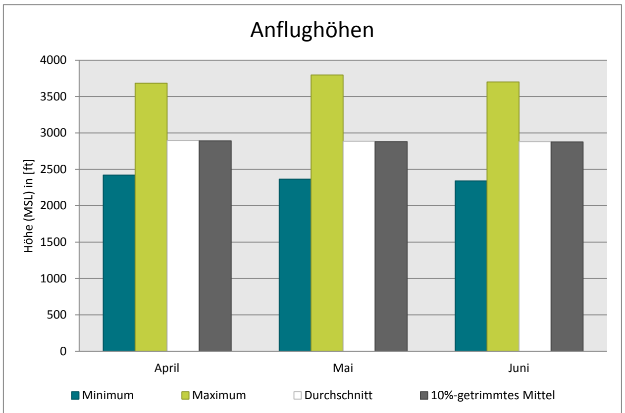
Abb. 8: Anflughöhen bei Betriebsrichtung 25
